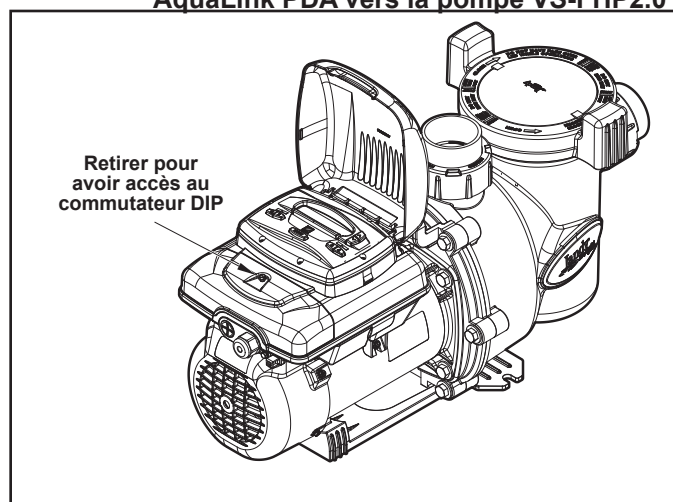
Figure 11. Couverture d'accès des commutateurs DIP du moteur de la pompe VS-FHP1.0
