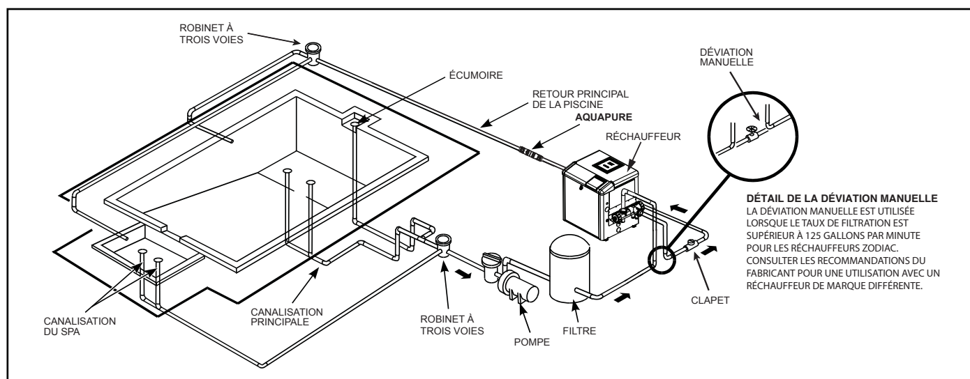
Figure 2. Installation typique de la tuyauterie
