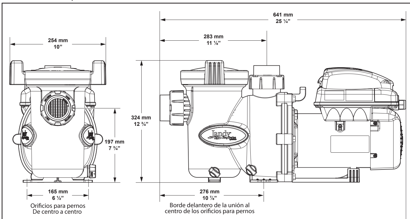
Figura 18. Dimensiones de la VS-FHP1.0
