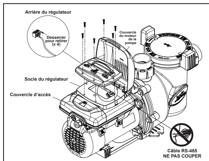
Figure 8. Débrancher le régulateur à vitesse variable (JEP-R) de la pompe VS-FHP1.0
