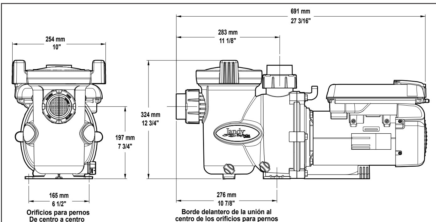
Figura 19. Dimensiones de la VS-FHP2.0
