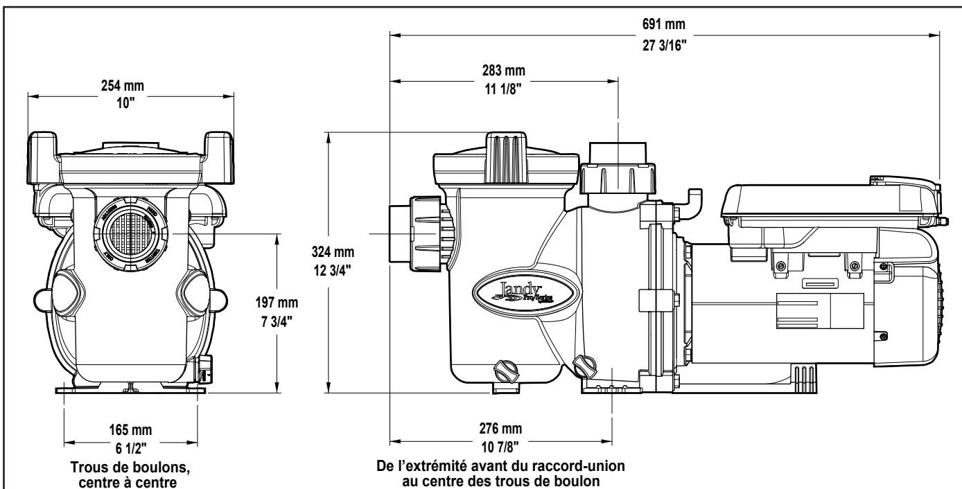
Figure 19. Dimensions de la VS-FHP2.0
