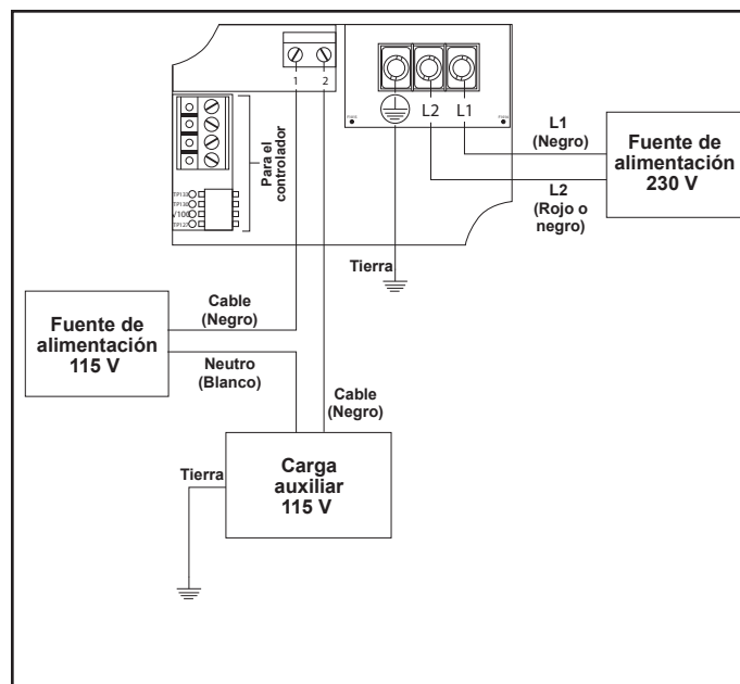
Figura 13. Diagrama de cableado de fuentes de alimentación separadas, carga auxiliar de 115 V
