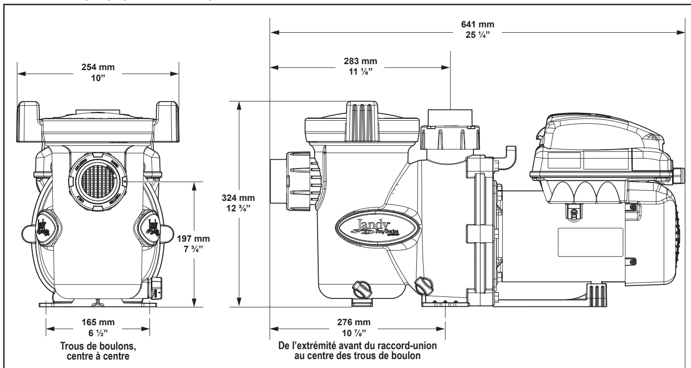
Figure 18. Dimensions de la VS-FHP1.0
