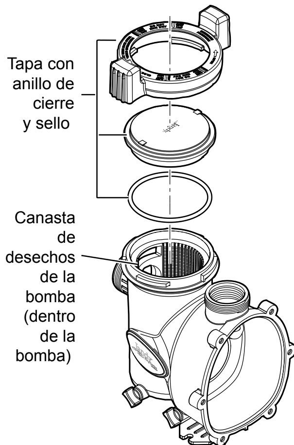
Figura 16. Plano de despiece de la bomba
