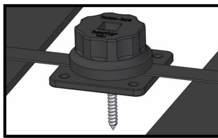
13. Soporte a Piso Instalado
