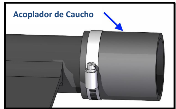
4. Acoplador de caucho
