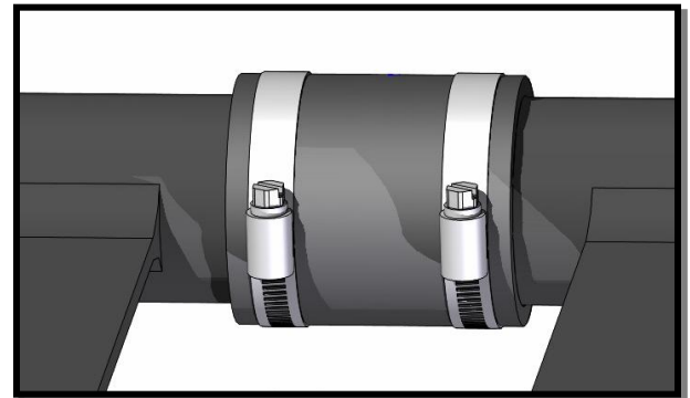
5. Acoplador de Caucho Instalado
