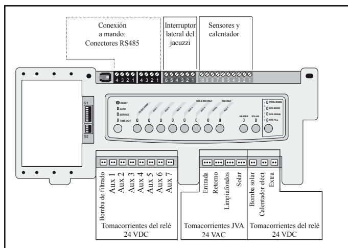
Figura 15. PCB con firmware REV N o posterior
